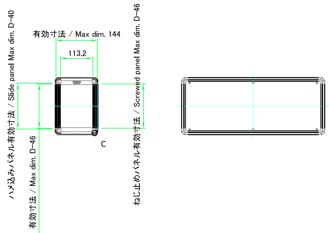
B-B ( 1 : 8 )
